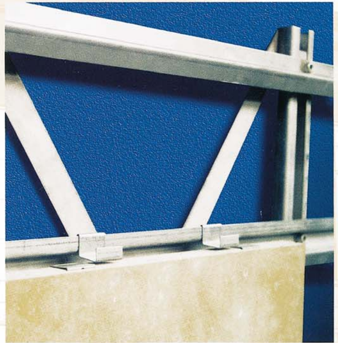
Détail du profilé en acier inoxydable et des clips de fixations
