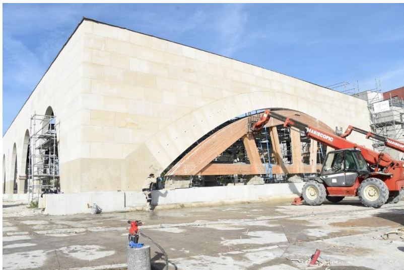
Enlèvement de la structure en bois de la façade Est, qui a permis la réalisation de l'arc en plein cintre avec la plus grande portée en Europe
